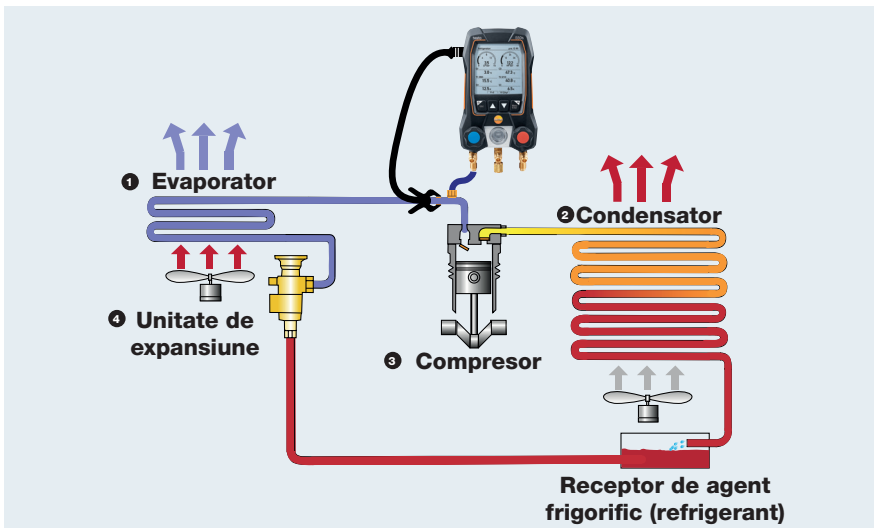
Determinarea nivelului de supraîncălzire la admisie
