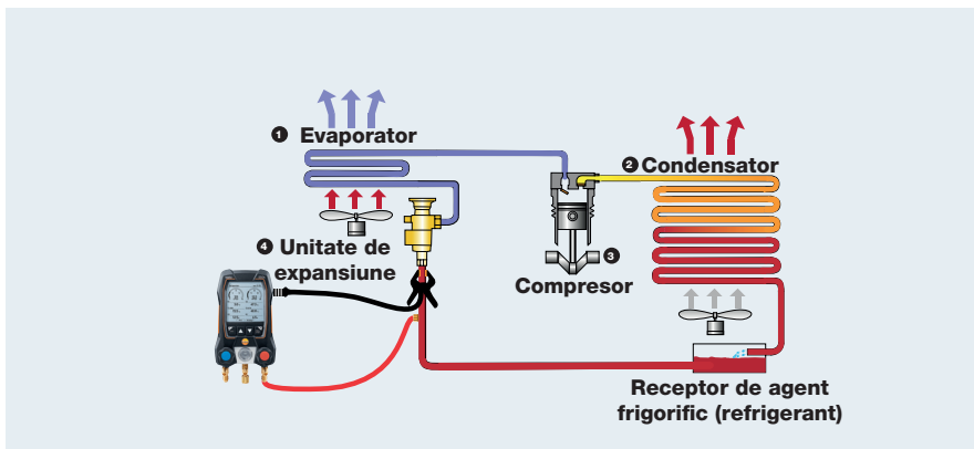
Determinarea subrăcirii înainte de etapa valvei de expansiune
