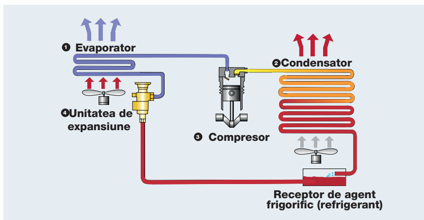
Circuit de agenți de refrigerare simplu, schematic
