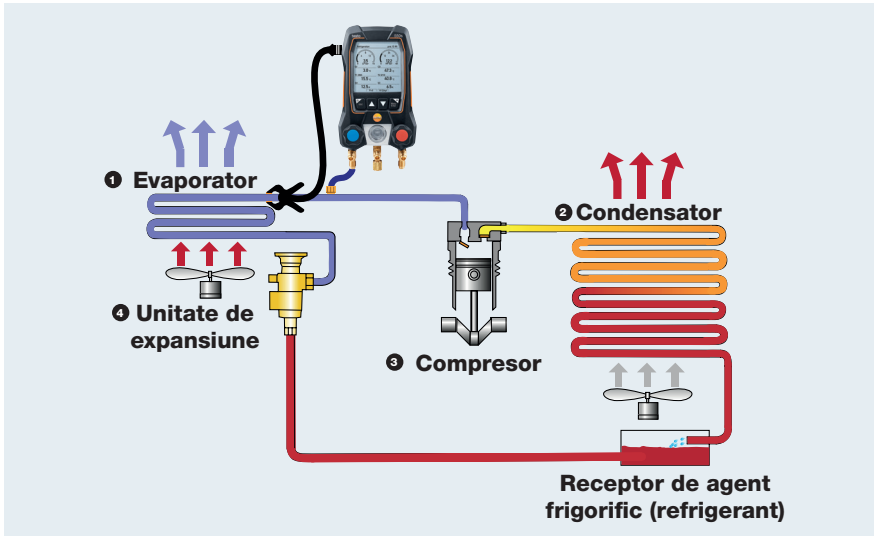
Determinarea cauzelor supraîncălzirii evaporatorului
